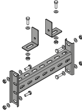
CCR/CR-UT Askı Takımı ("T" civatasız)
